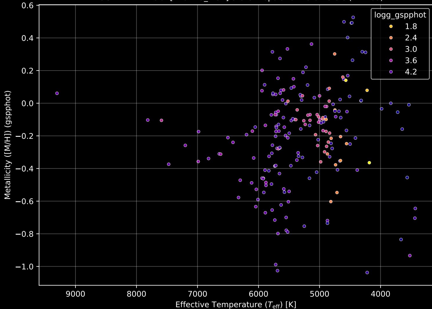
APOGEE DR17 Field: [246+49_MGA] Stellar Population Parameters (n= 203)
